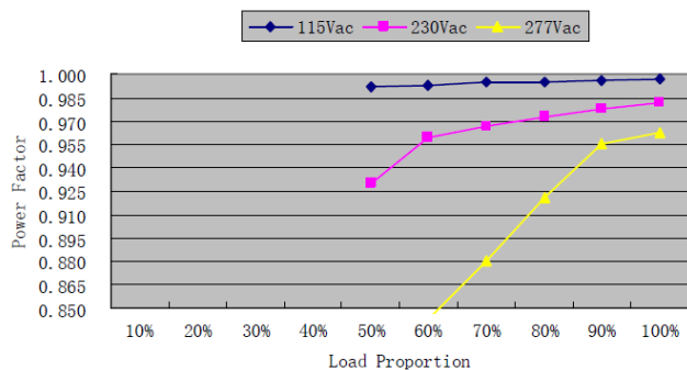
GLSV-100B036
