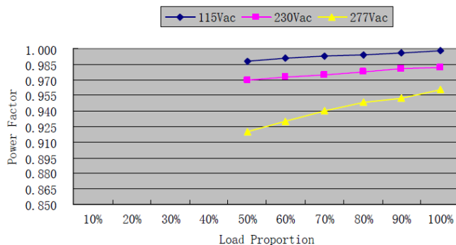
GLSV-100B048
